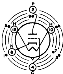
INDEX - LARGE LUG ● - SHORT PIN; IC - DO NOT USE
