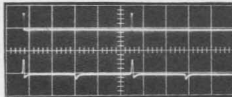
V106, pin 2, 20v/cm, 2 \mu sec/cm. V102, pin 6, 20v/cm, 2 \mu sec/cm.
